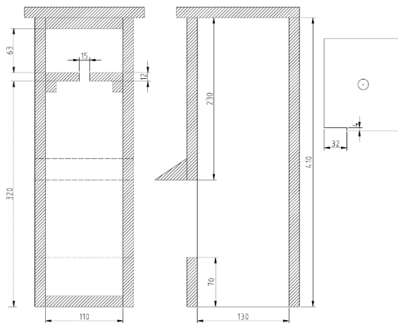
Ontwerp van het nestkastje
